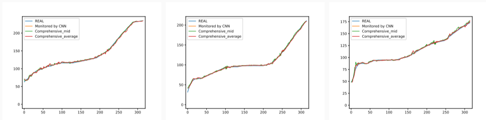
Figure 28: 真实磨损量、CNN 监测值、基于平均数和中位数的磨损量修正结果
